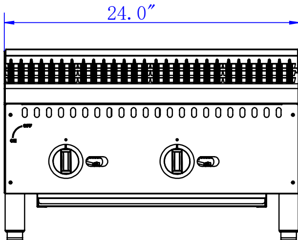
HSD-SG-24
